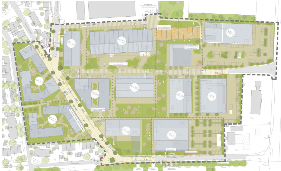
Abb. 8: Auszug aus der Erschließungsplanung – Lageplan Verkehrsanlagen, Stand 17.12.2021, WipflerPLAN•Köpf Planungsgesellschaft mbH auf Basis der Freianlagenplanung Jühling Köppel Landschaftsarchitekten, o.M.
